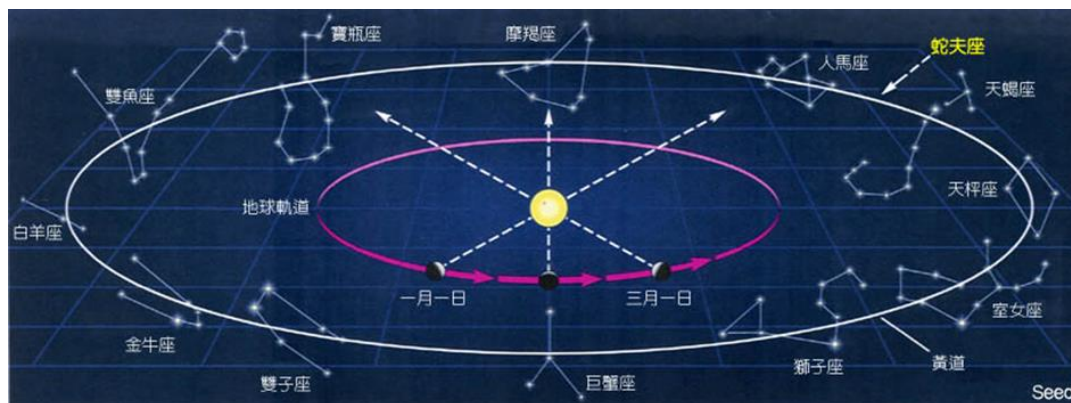
圖：黃道上的星座
